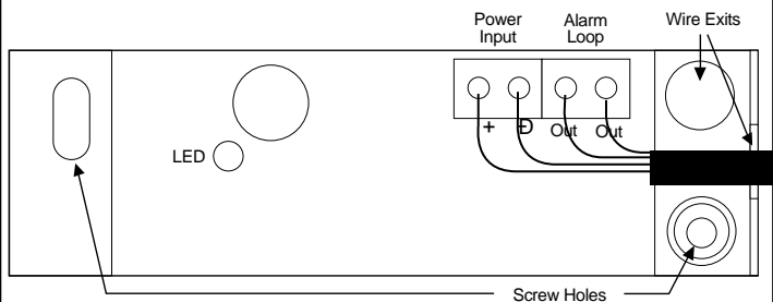
5422 Wiring Guide
